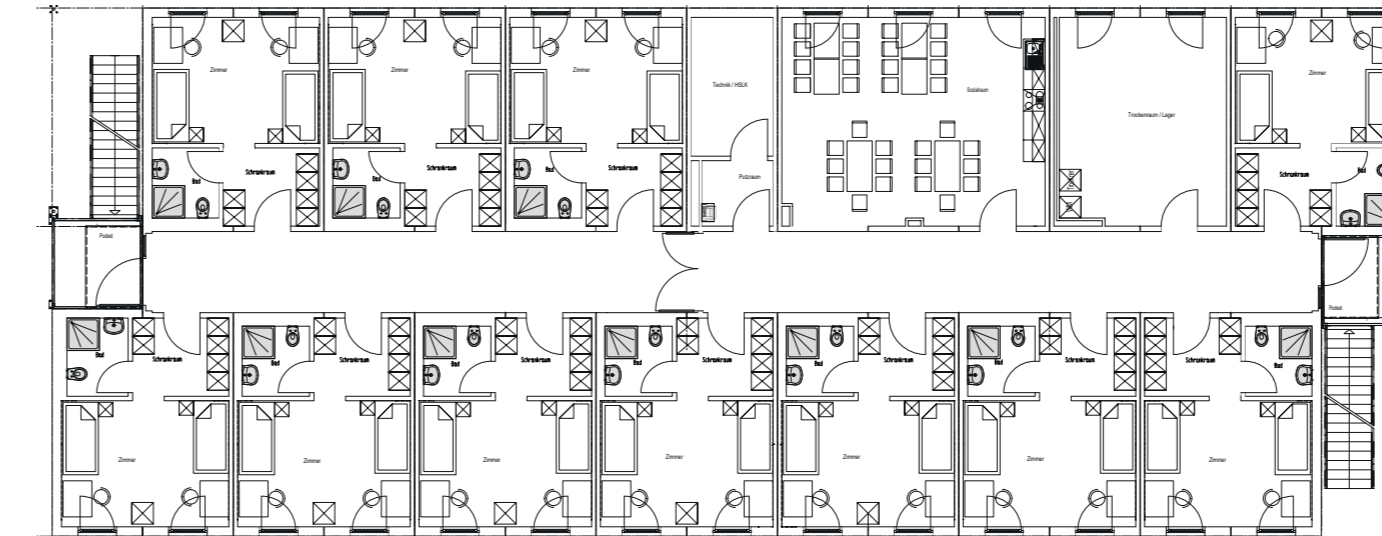
| Grundrissausschnitt Bereitschaftspolizei Dachau
