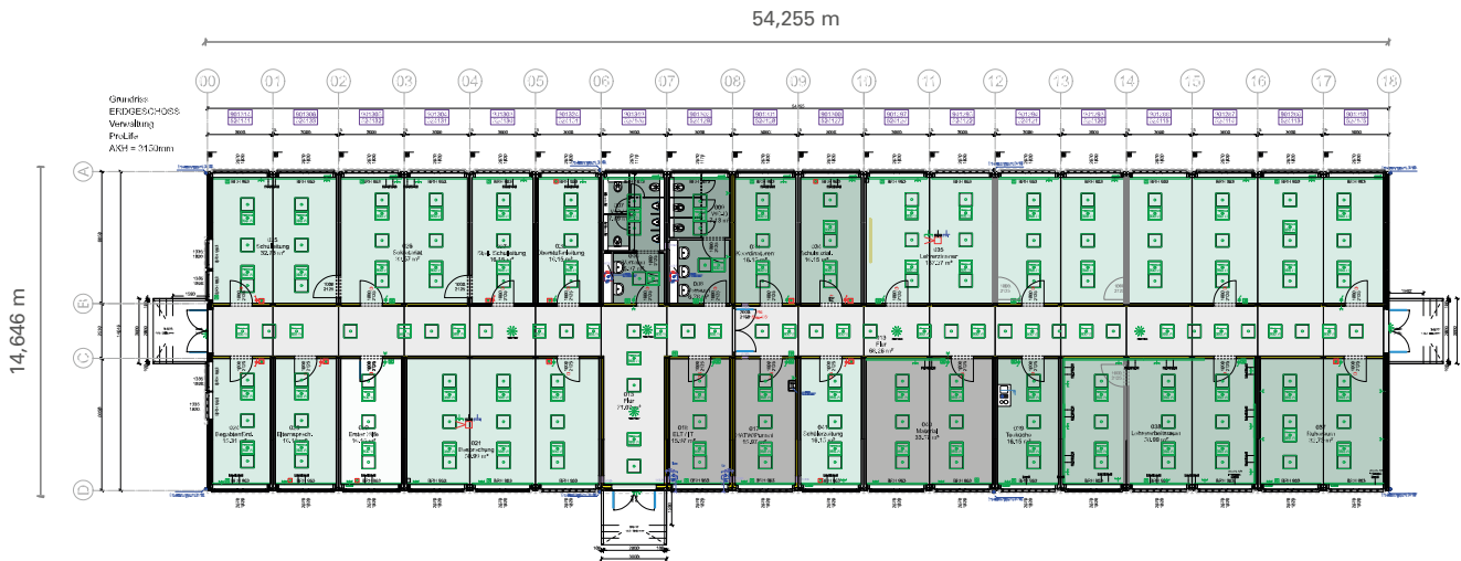
Grundriss Erdgeschoss
