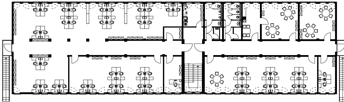
Grundriss Obergeschoss
