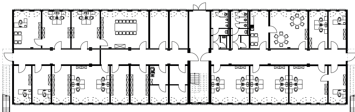
Grundriss Erdgeschoss
