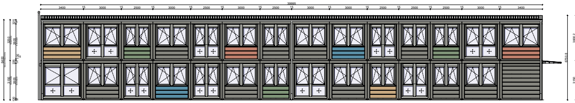
Ansicht Nord-West
