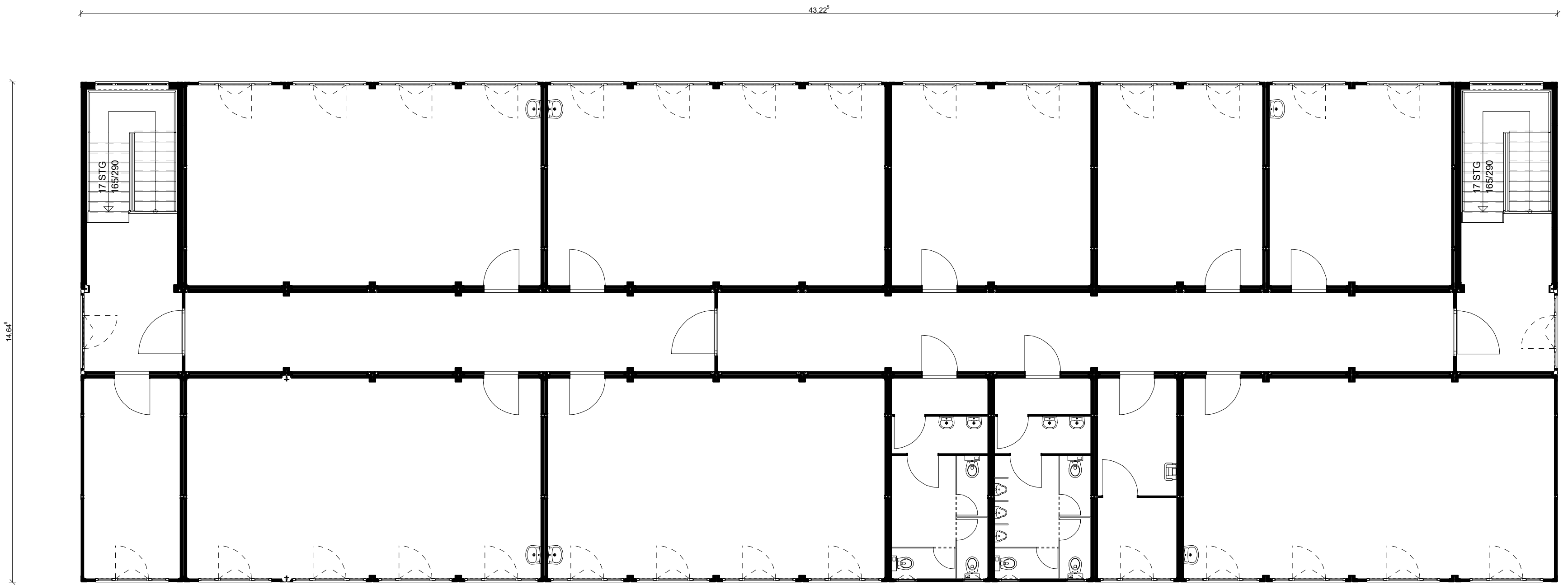
Grundriss OBERGESCHOSS
